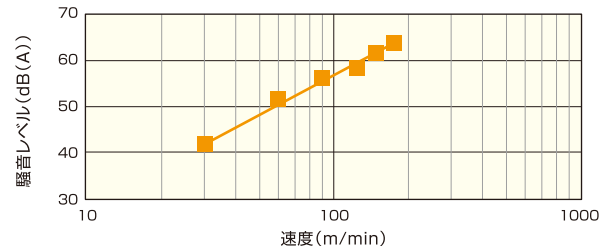
騒音レベル測定
