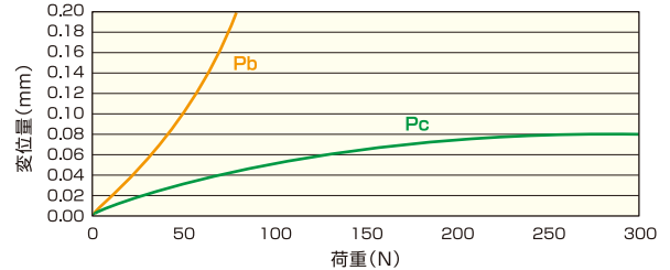
剛性試験データ
