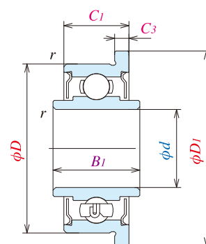
シールド形 Shielded type ZZ
